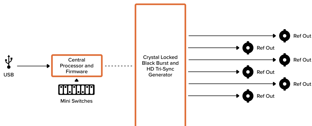
Схема соединений Mini Converter Sync Generator
