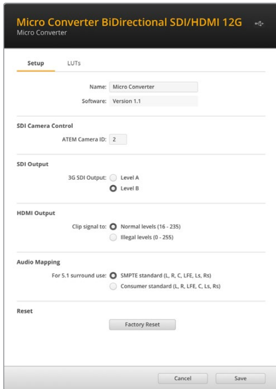
Optionen für die Einrichtung des Micro Converter BiDirectional SDI/HDMI 12G
